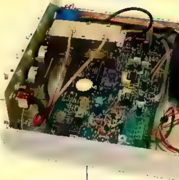
Het interieur van de analyzer
